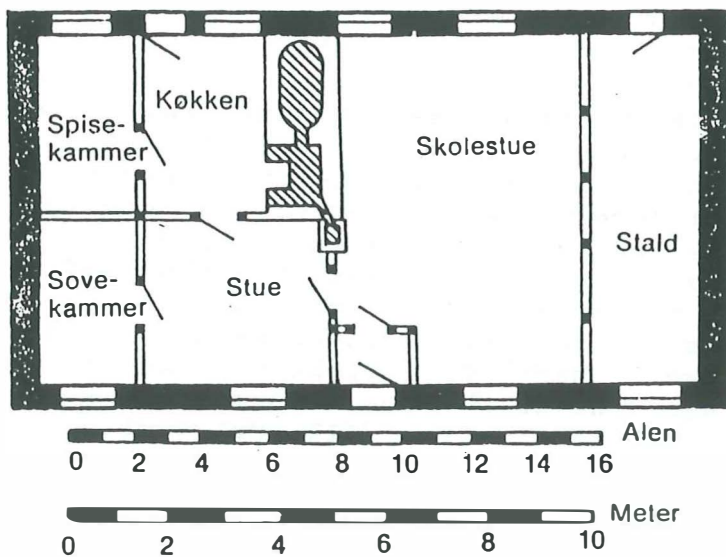
Rytterskolernes grundplan.
